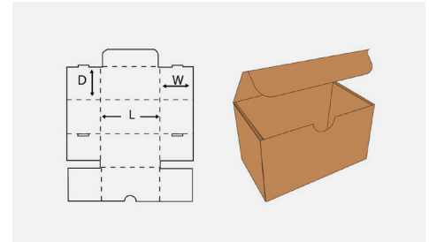
R.E.T.T. (Econo Roll End Tuck Top)
