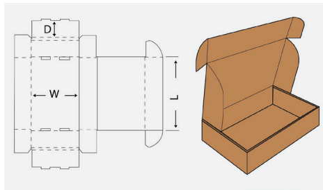
R.E.L.F. (Roll End Lock Front)
